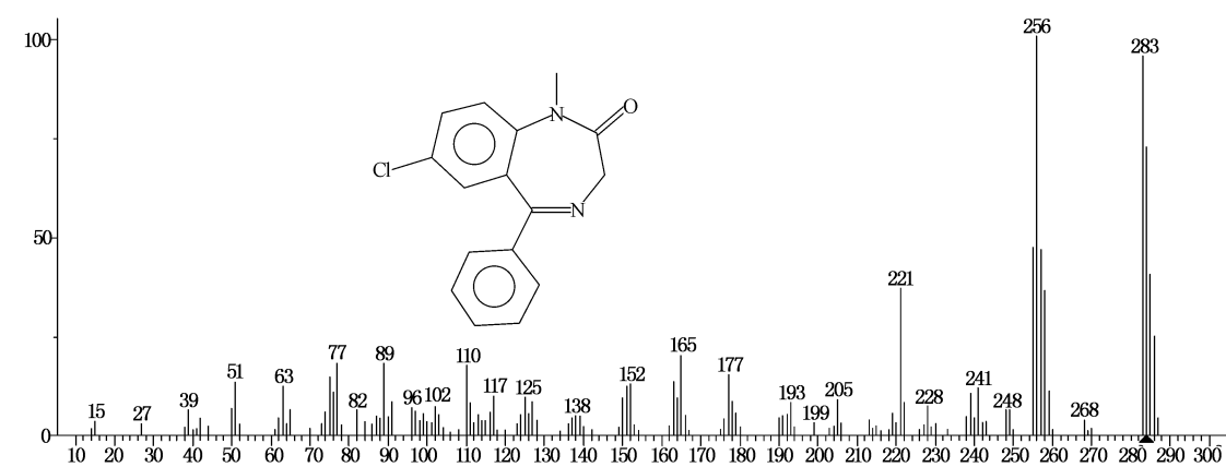
图 B.2 地西洋质谱图
