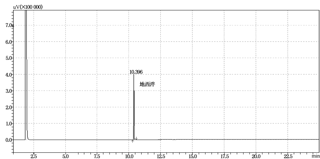
图 B.1 地西洋气相色谱图
